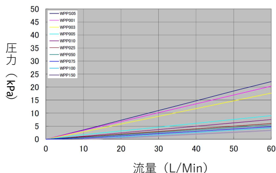
【流量特性 (@ 250mm)】
